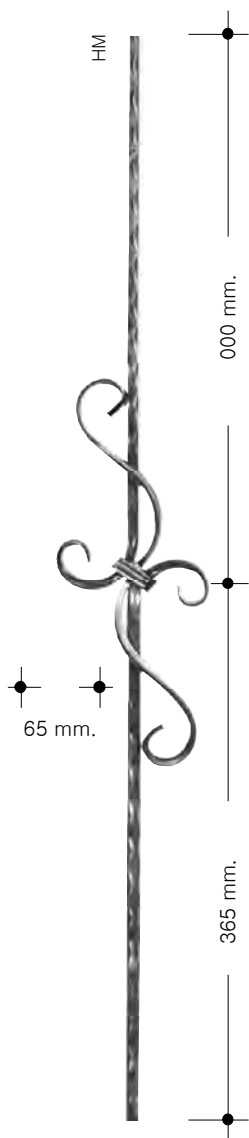
P-1701HM 1.550 kg.-3.416 lbs. Dim.140 x 900 mm. 5 4 / 8 x 35 7 / 16
