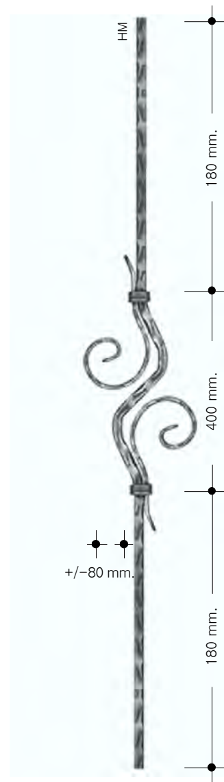
P-4901/A HM 1.600 kg.-3.526 lbs. Dim.150 x 900 mm. 5"7/8 x 35"7/16
